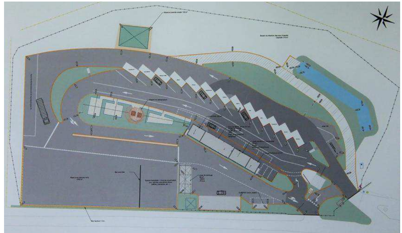
Le plan de la future déchetterie. La zone en gris foncé correspond à l'emprise actuelle du site. Le projet du Sytevom inclut également la création d'un espace pédagogique, avec un observatoire, pour accueillir notamment des scolaires. Document Sytevom
